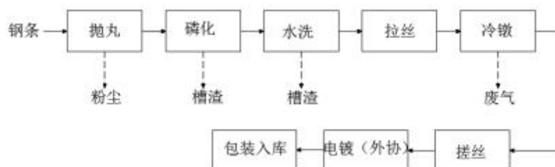
图 2-1 本项目生产工艺流程及产污环节
