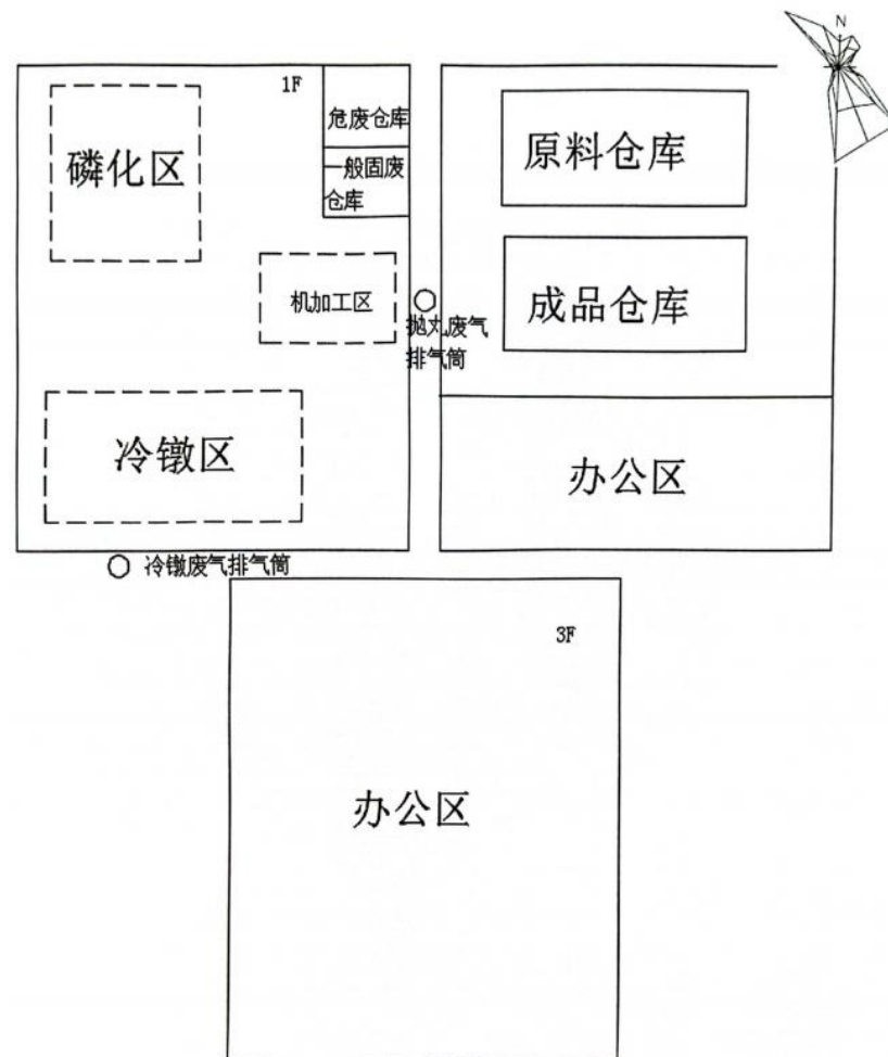
图 3 项目平面示意图
